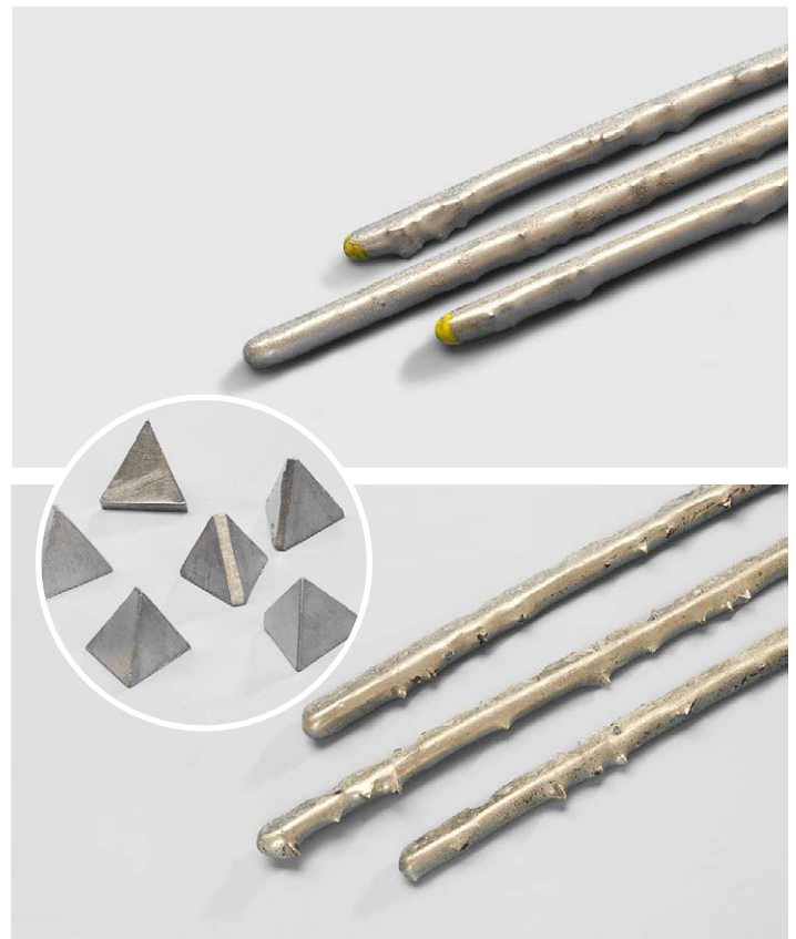
Top: WokaDur SA 100-Ni. Bottom: WokaDur SA 100-Ni-T. Inset: Tetrahedral carbides used in WokaDur SA 100-Ni-T.
