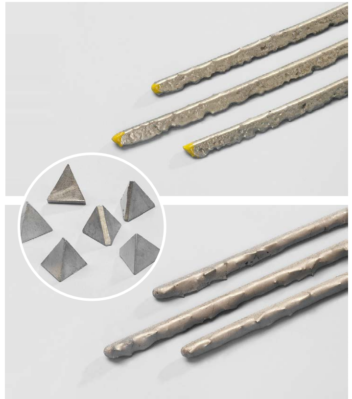
Top: WokaDur SA 100. Bottom: WokaDur SA 100-T. Inset: Tetrahedral carbides used in WokaDur SA 100-T.
