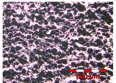
Metco 601NS 宏观硬度 (R15Y) : 62.5 - 70.5 易磨损相+孔隙率 54.5 - 57
