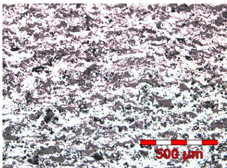
Metco 313NS 宏观硬度 (R15Y) : 65 - 75 易磨损相+孔隙率 45 - 50
