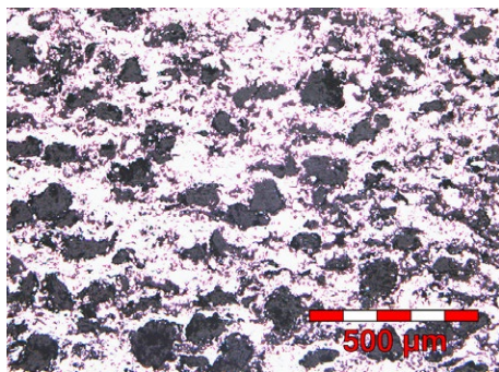
Metco 320NS 宏观硬度 (R15Y) : 56 - 62 易磨损相+孔隙率 51 - 57
