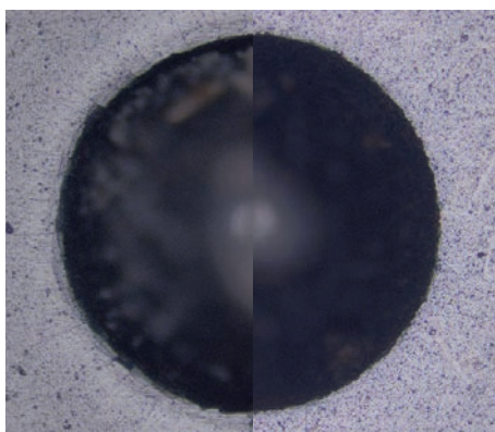
BALINIT® ALCRONA PROとBALINIT® ALCRONA PRO ADVANCEDの比較: 優れた母材表面硬度による弾性変形の減少
