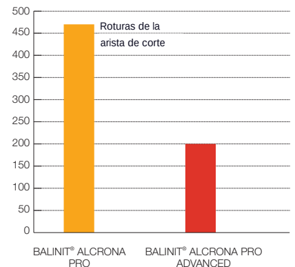
Desgaste de la superficie lateral (µm) tras 25.000 golpes
